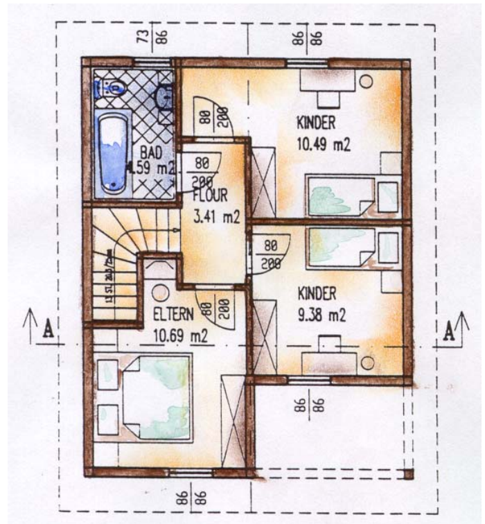
OBERGESCHOSS
